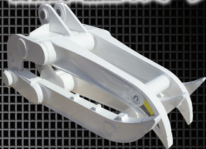
機械式2点止めフォーク
