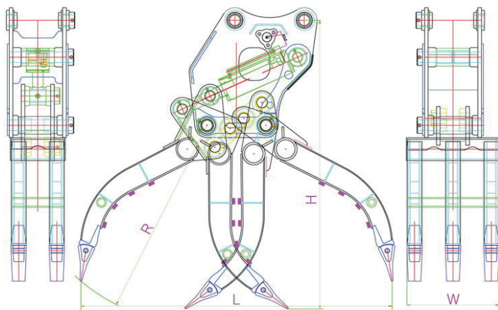
■油圧式フォークグラップル 仕様
